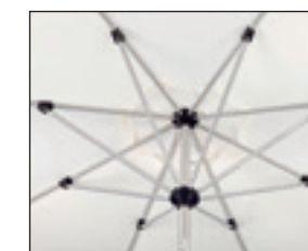
Gestänge mit 20 mm starken, runden Streben. Alle Kunststoffteile sind schwarz.
